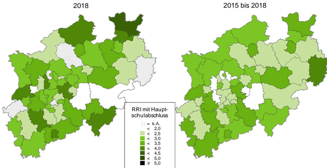
Abbildung C-2: RRIs geflüchtete vs. nichtgeflüchtete Abgängerinnen und Abgänger mit Hauptschulabschluss von allgemeinbildenden Schulen in den Kreisen und kreisfreien Städten NRWs (Abgangsjahr 2018 sowie Abgangsjahre 2015 bis 2018 für Abgängerinnen und Abgänger mit vs. Abgängerinnen und Abgänger ohne einer Staatsangehörigkeit mit im Jahr 2018 überwiegenderem Geflüchtetenanteil im Schulbesuchsalter)
